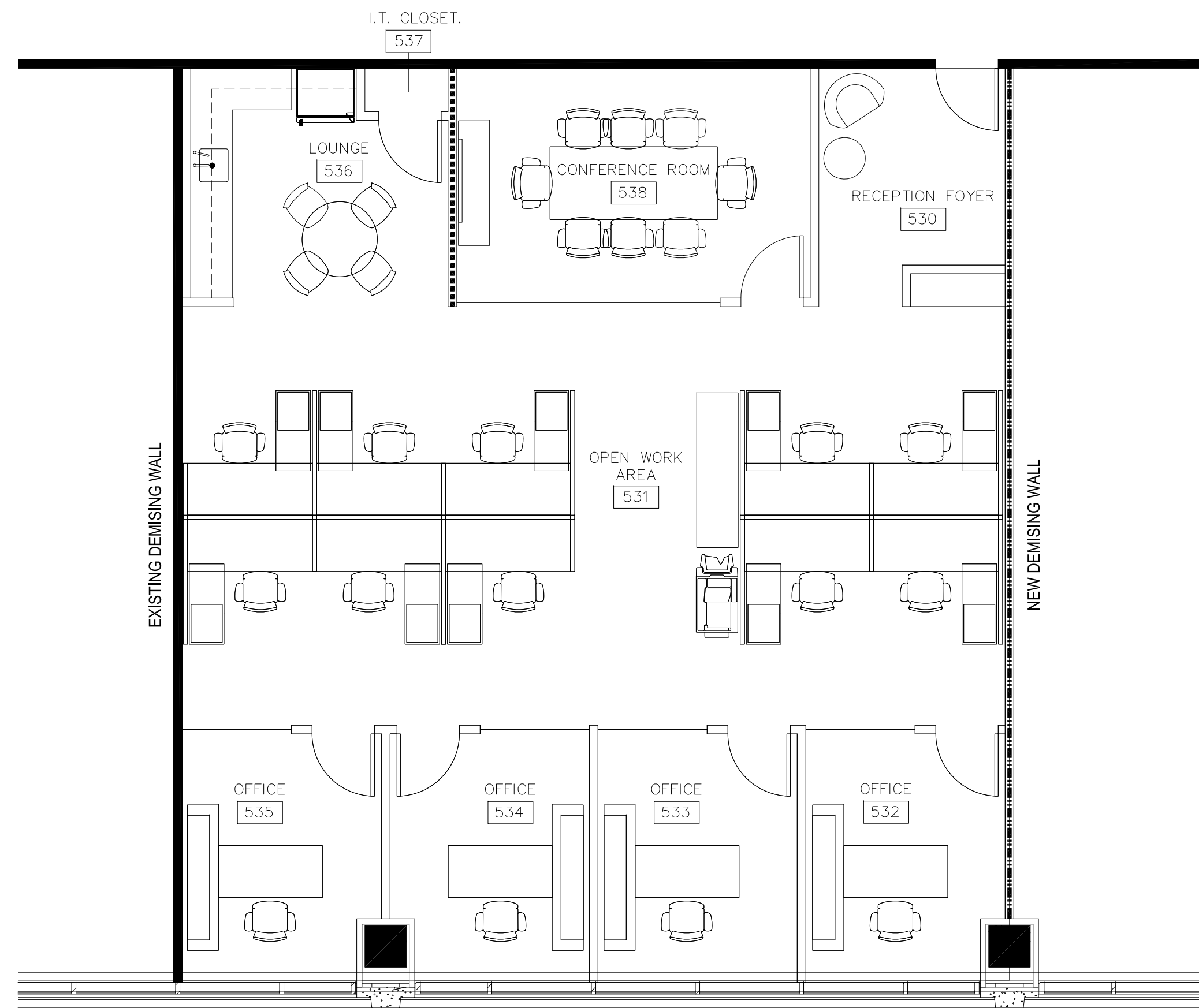
N SPACE PLAN SCALE: \frac{3}{16}'' = 1'-0''
