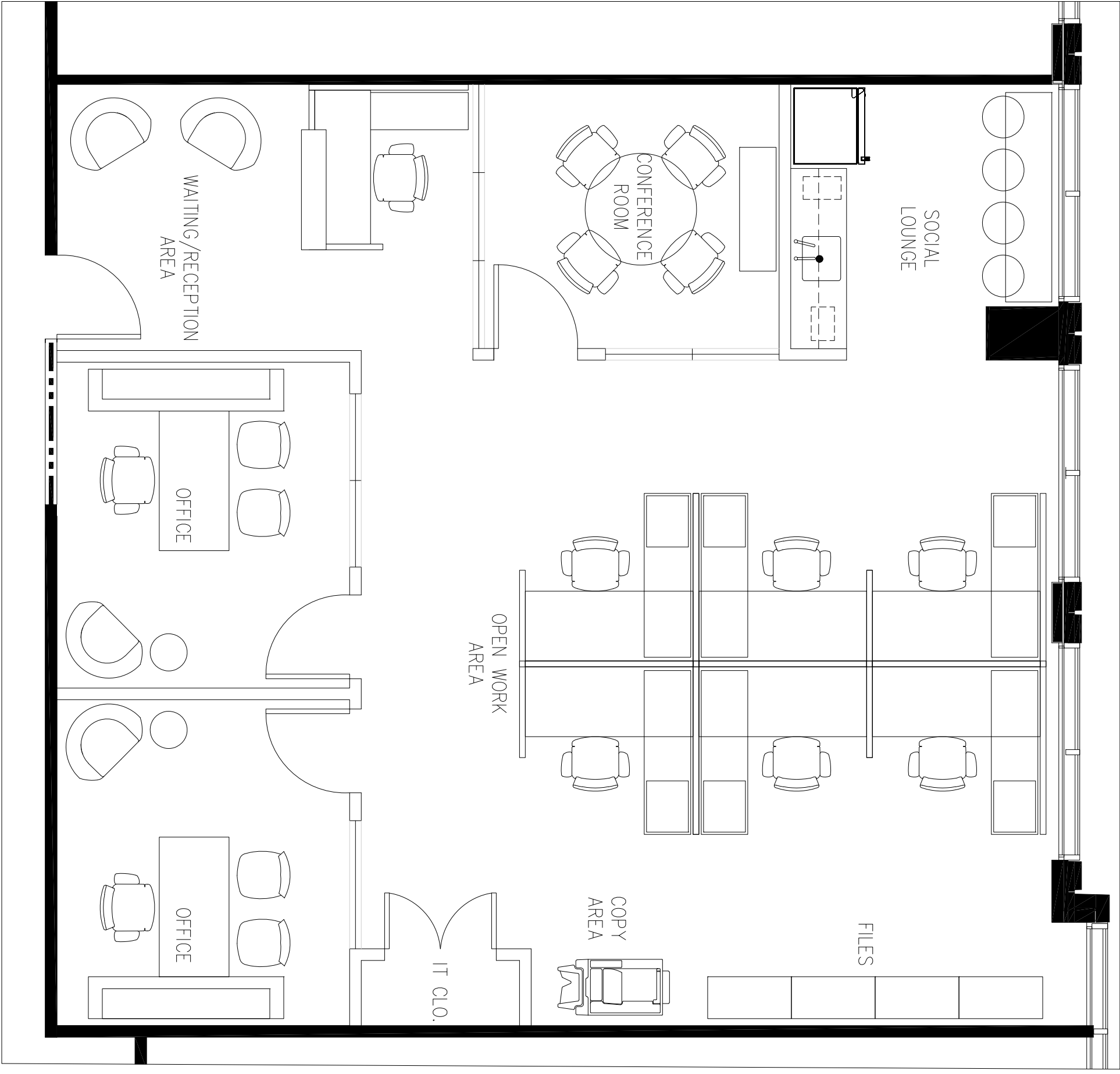
SPACE PLAN SCALE: \frac{1}{4}''=1'-0''
